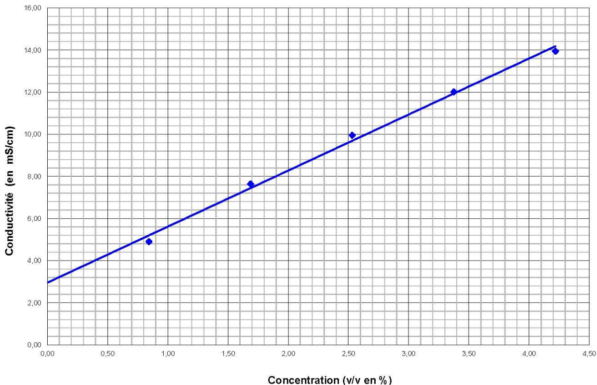
Courbe de conductivité à 25°C du CAM 4102 - V1 Courbe réalisée avec une eau de dureté = 21°f avec le conductimètre WTW Cond 3110
